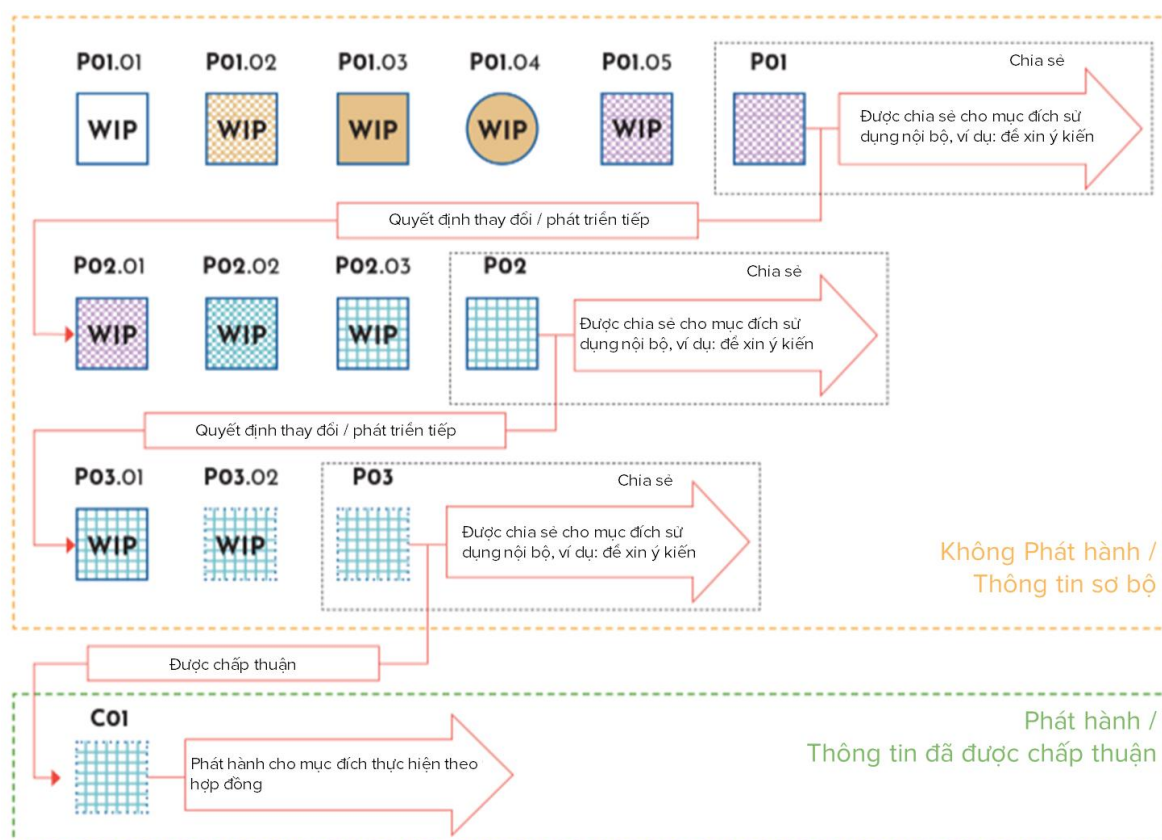
Hình 3.7 Ví dụ về chuyển đổi mã kiểm soát phiên bản đến giai đoạn phát hành
